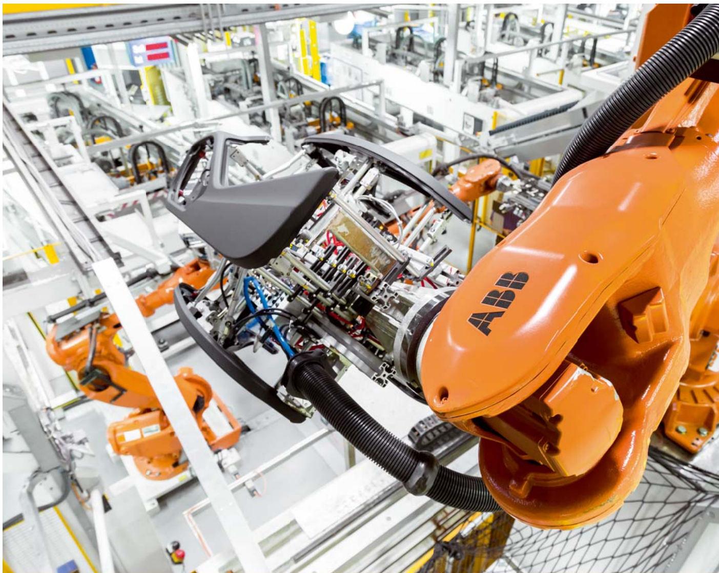
Die Anlage für das Kaschieren und Umbugen der Türinnenverkleidungen erstreckt sich über zwei Ebenen.
